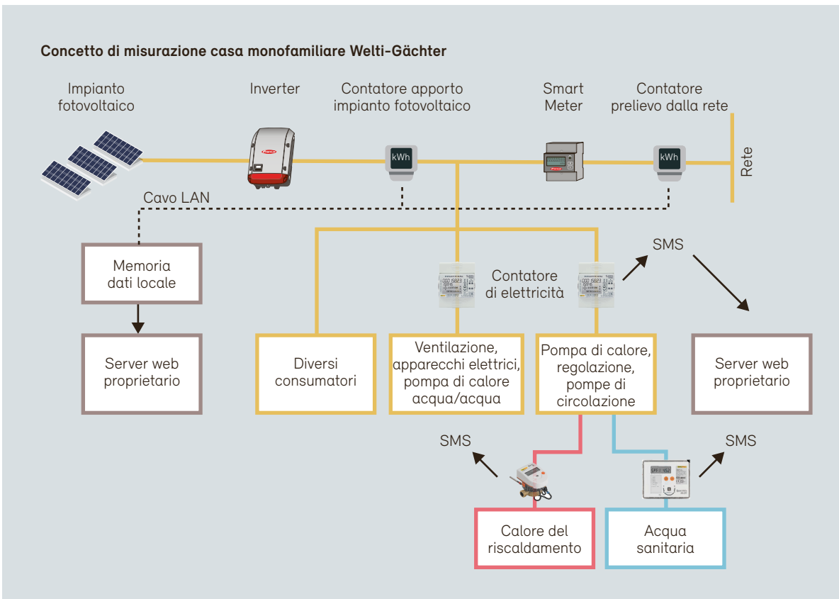
Figura 2: La casa Minergie-A a Oberriet è una casa energia-Plus e ciò è confermato dal monitoraggio.
